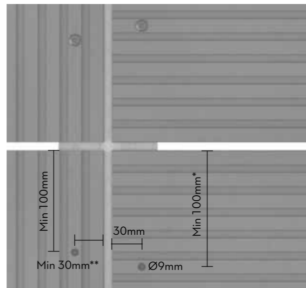
Fig. 3. Cembrit Patina Inline edge distances.
